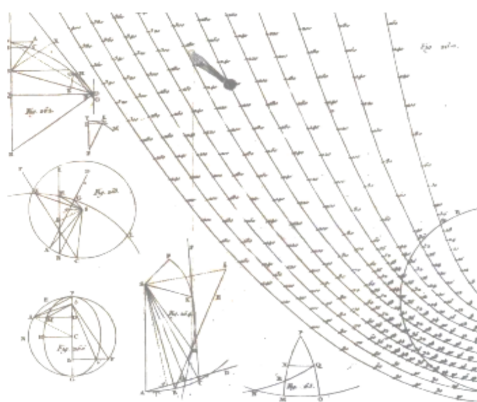
astronomija
